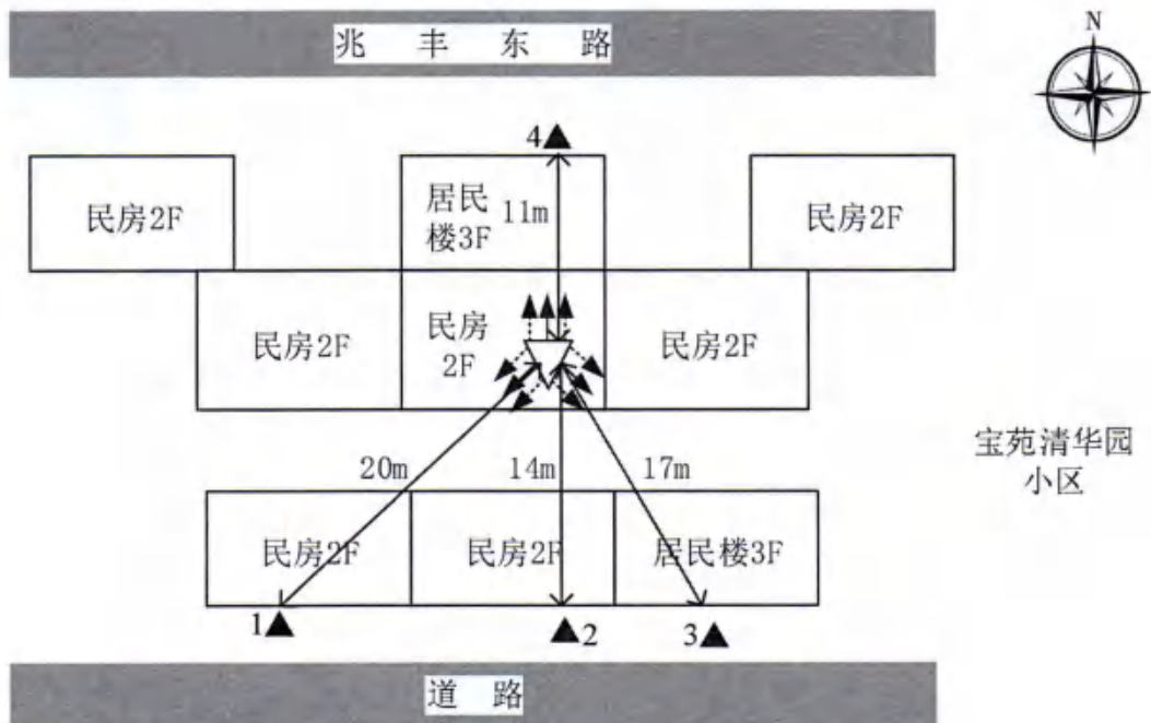
基站电磁辐射环境检测点位示意图
