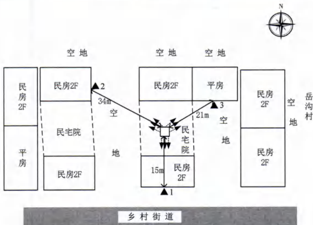
基站电磁辐射环境检测点位示意图
